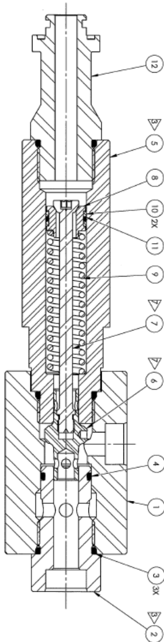
SECTION A-A
